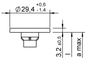
Scheiben-/Tellerkopf III – mit und ohne Fräskanten
