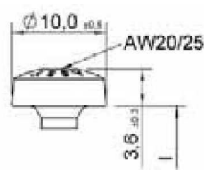
Tête Pan head
