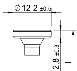
Flachkopf
