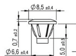
Top head II – Z i bez soczewki
