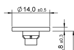
Scheiben-/Tellerkopf III – Ausführung mit und ohne Fräskanten
