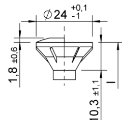
Fräskantensenkkopf – mit und ohne Linse
