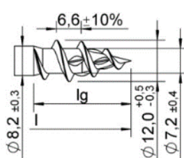
grubozwojny II
