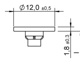
Scheiben-/Tellerkopf III – mit und ohne Fräskanten
