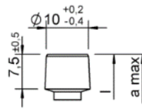
Łeb walcowy
