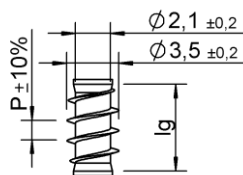
Unterkopfgewinde Lg2 < 4 x d, P = 1,6; 2,2; 3,2
