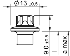
Außensechsrundkopf – mit und ohne Kragen/Scheibe
