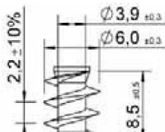
Filetage sous tête
