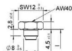
Tête Kombi
