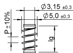
Unterkopfgewinde Lg2 < 4 \times d P = 2,2; 3,1; 4,4
