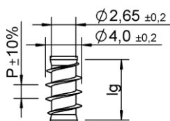
Unterkopfgewinde Lg_2 < 4 \times d , P = 1,8
