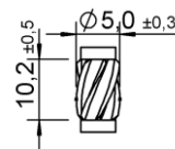
Schaftfräser
