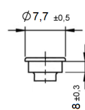
Stufenkopf
