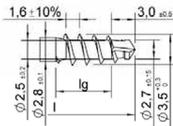
ASSY plus spéciale
