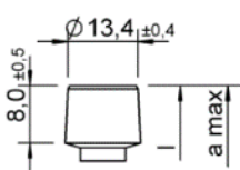
Łeb walcowy
