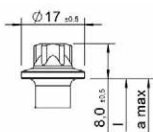
Tête hexalobulaire
