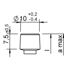
Zylinderkopf
