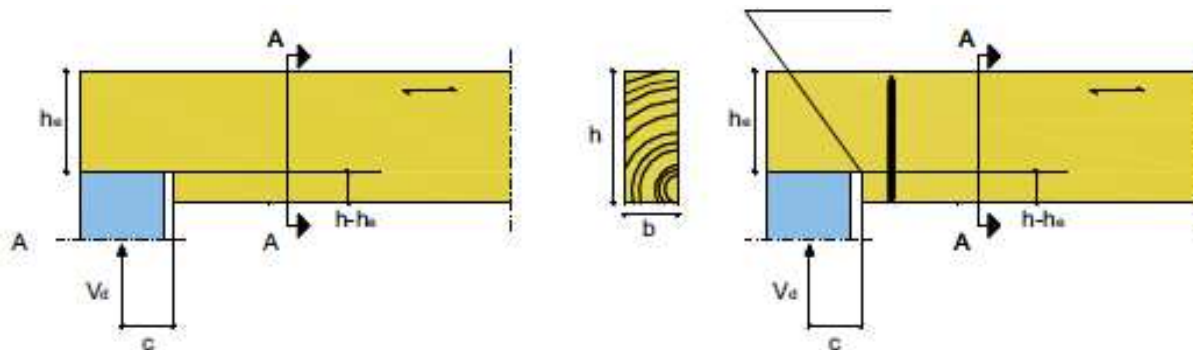
Figure 3.2 : Exemple de renforcement d'une encoche en cas de traction perpendiculaire au fil
