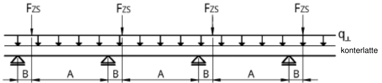
Figure 5.5 : Contre-latte continue soumise à une charge linéaire constante sur la surface du toit q_{\perp} et à des charges isolées provenant des vis sollicitées en traction F_{zs}
