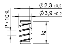
Unterkopfgewinde Lg2 < 4 x d, P = 1,6; 2,0
