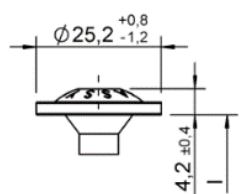
Łeb podkładkowy powiększon / talerzykowy I
