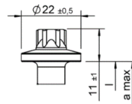
Łeb zewnętrzny Torx – z i bez kołnierza / podkładk
