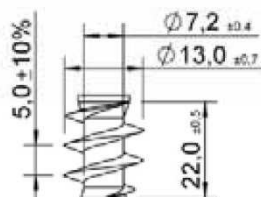
Filetage sous tête
