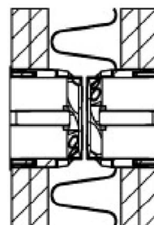
Beidseitiger Einbau Mehrfachanordnung
