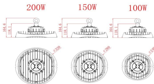
Abb. 2: Seitenan- und Draufsicht der EGH mit Maßen in mm.
