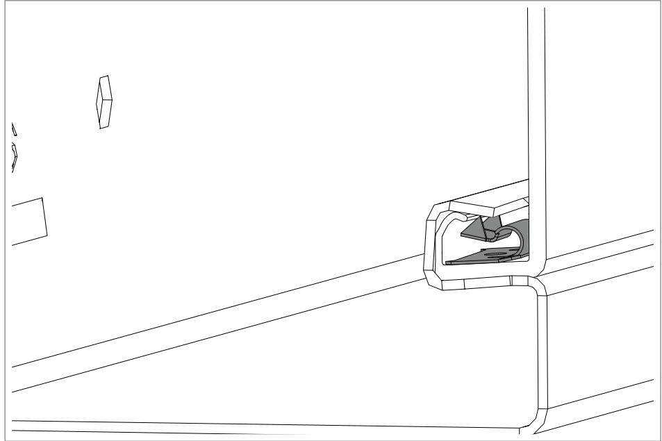
Abb. 2: Rastklammern montieren
